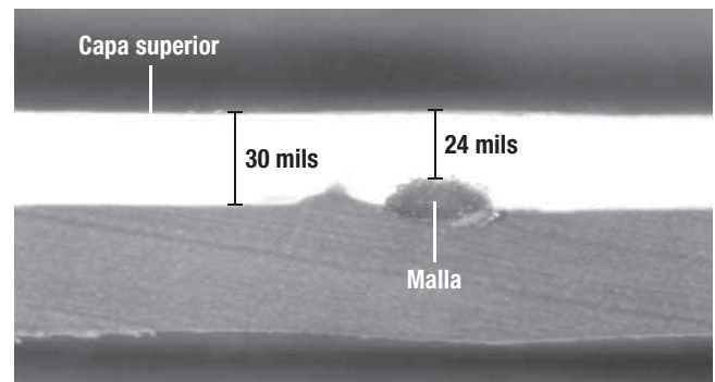
SECCIÓN TRANSVERSAL DE LA MEMBRANA DE TPO
